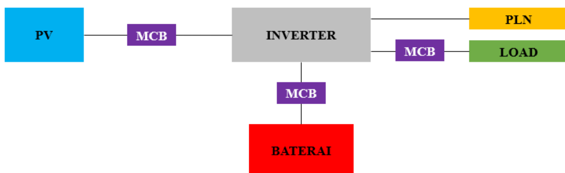
Gambar 7. Desain Instalasi Sistem PLTS
