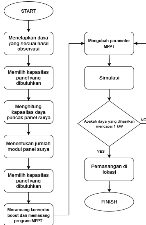
Gambar 4. Bagan Alir Rancang Bangun TTG
