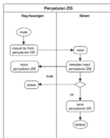
Gambar 7. Actifity diagram penyaluran ZIS
