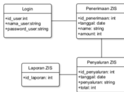
Gambar 9. Class diagram sistem informasi
