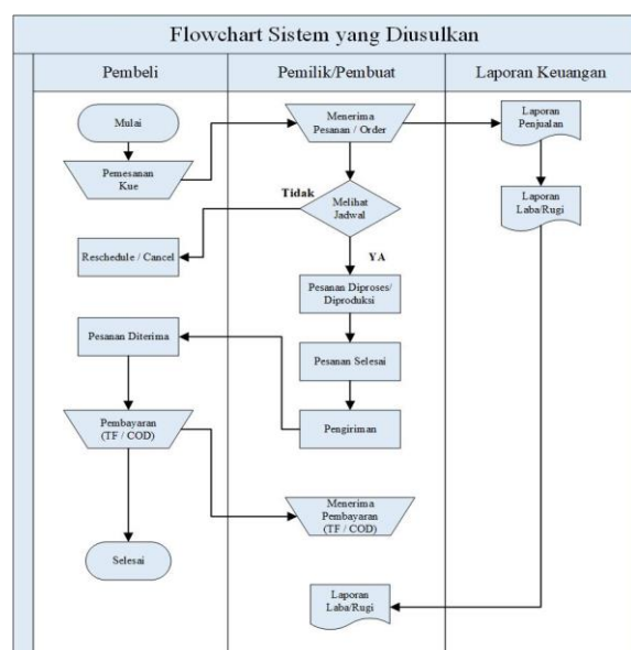
Gambar 2. Flowchart Usulan Laporan Keuangan Lucyake
