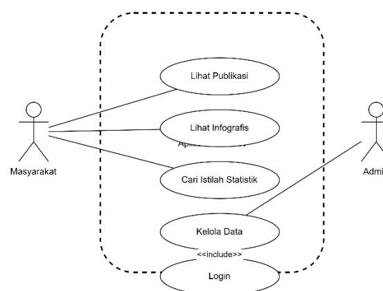
Gambar 1. Use Case Diagram Aplikasi MEDIAN
