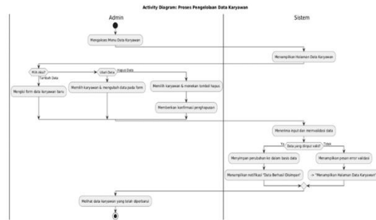
Gambar 1 Activity pengelolaan karyawan
