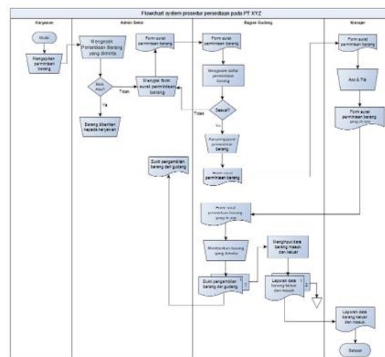
Gambar 3. 3 Flowchart sistem persediaan yang berjalan
